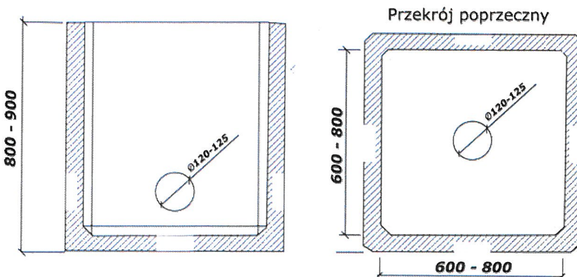
Rys. Studnia kablowa.
