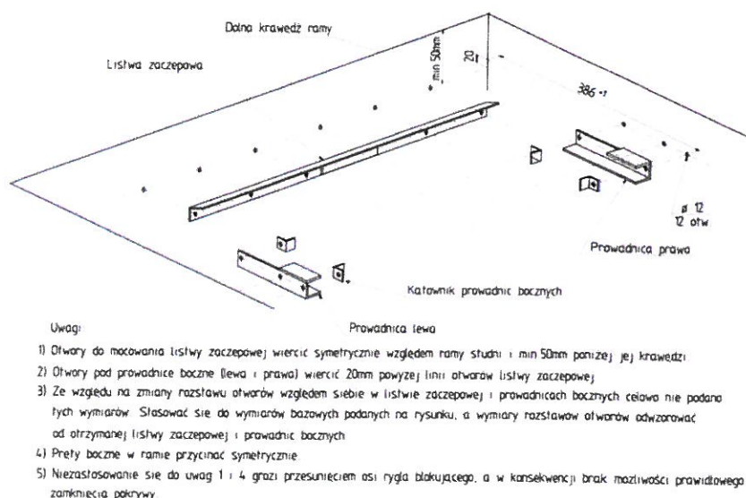
Rys. Schemat wykonania zamknięcia studni
